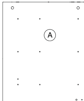
F17959 580x478x18mm
